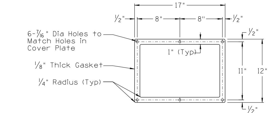
NEOPRENE GASKET
