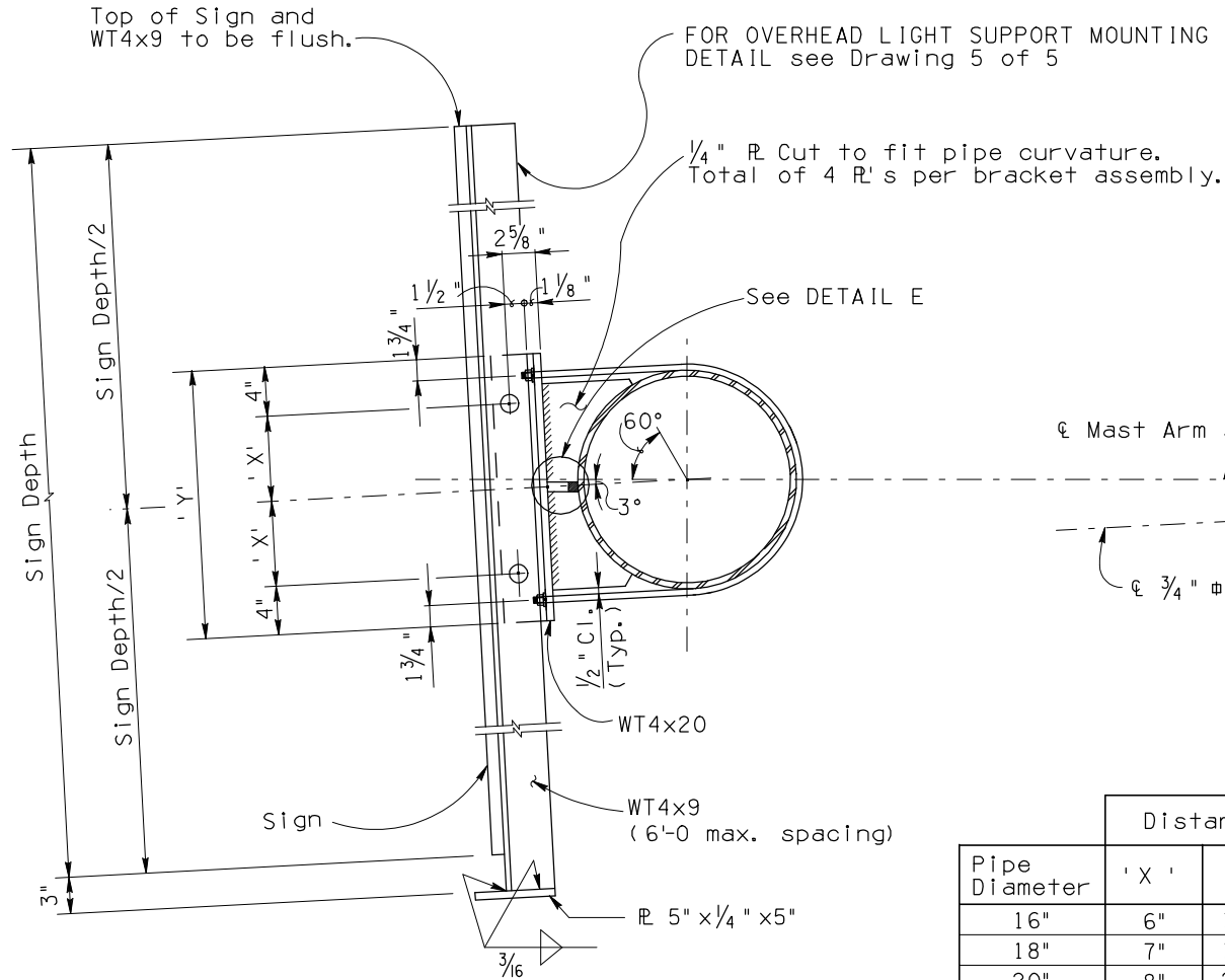
ELEVATION C-C
